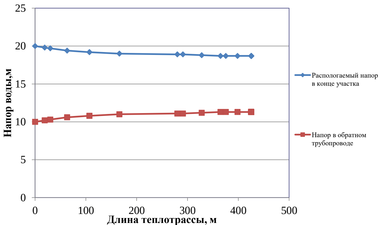
Рисунок 2.4 – Пьезометрический график тепловой сети Котельной с. Буготак от котельной до пер. Центральный, 34
