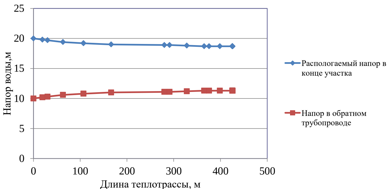
Рисунок 2.3 – Пьезометрический график тепловой сети котельной с. Буготак
