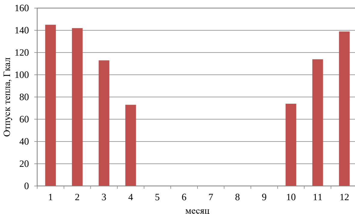
Рисунок 1.3 – Оптимальный температурный график отпуса тепловой энергии для котельной с. Буготак
